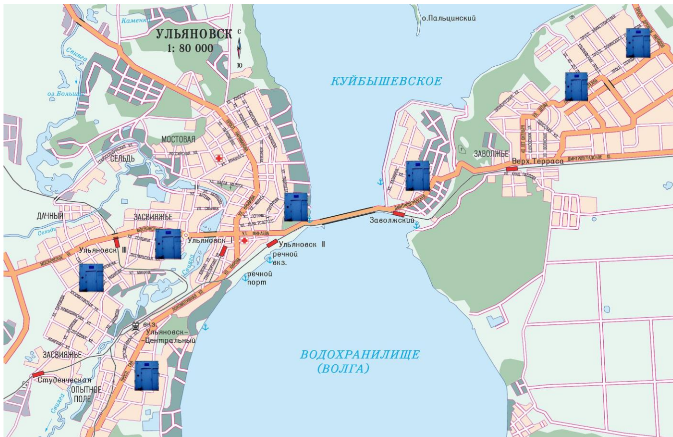
Карта-схема 1. Расположение стационарных постов наблюдений за загрязнением атмосферы (ПНЗ) в г. Ульяновск
