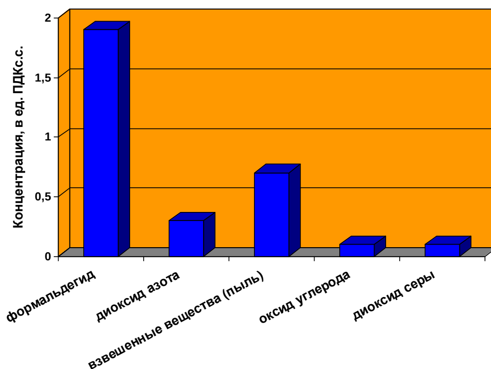
Уровни загрязнения атмосферы г. Сенгилей
